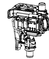
VALVOLA DRENAGGIO BACINELLA Da collegare al motore aspirante con separatore integrato.
